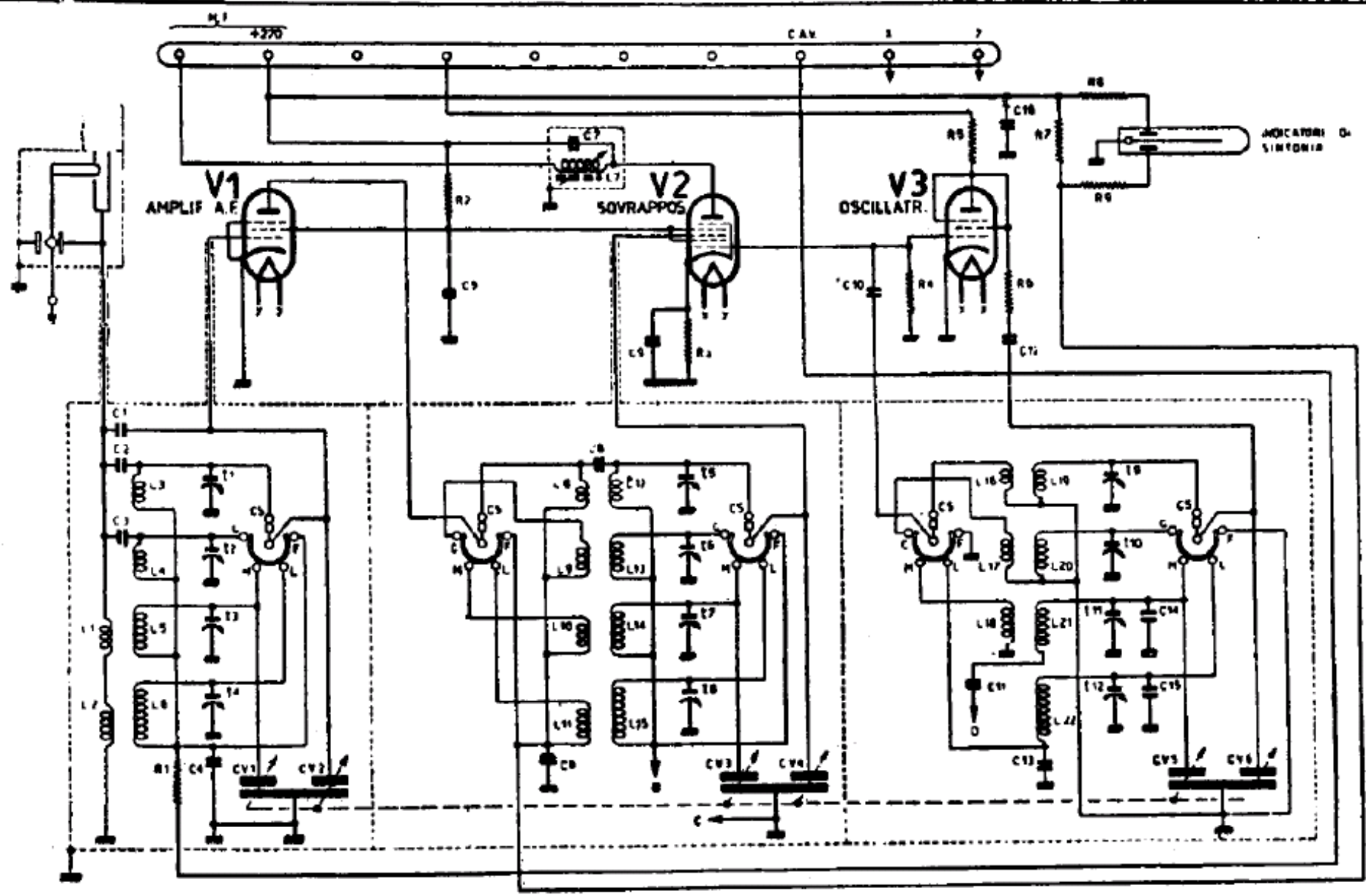
PHONOLA (S. A. FIMI). — Mod. 617. — Complesso A. F. — Serie ultraconvert. — Produzione 1938-39 — Media frequenza: 470 kHz
